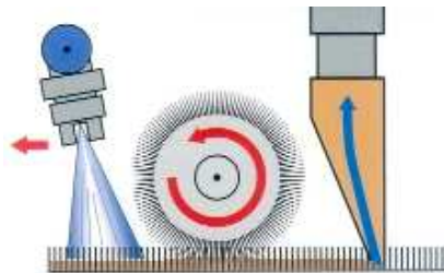
Nettoyage par injection extraction avec brosse tournante
